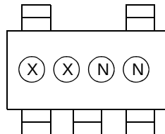
5-Pin SC-70/SC-70R
