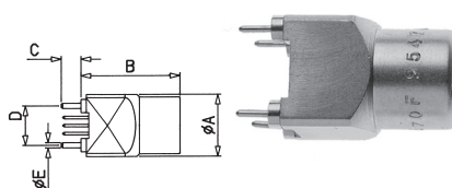
EZ : PCB
