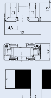
Solder pads / Anschlussflächen
