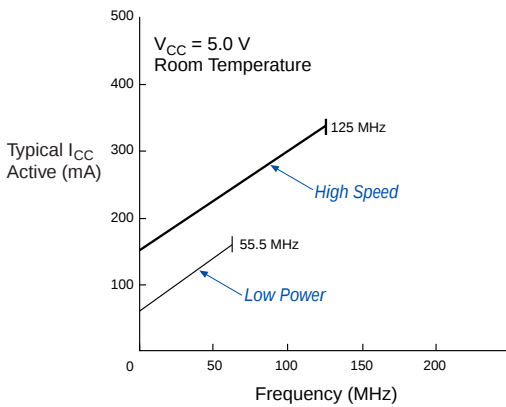
EPM7128E
