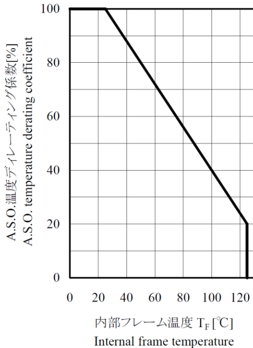
STR-X6759B A.S.O.温度ディレーティング係数曲線 A.S.O. temperature derating coefficient curve
