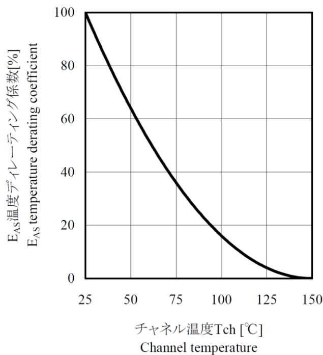
STR-X6759B アバランシェ・エネルギー耐量 ディレーティング曲線 Avalanche energy derating curve
