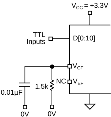
Figure 14. VCF/VEF Biasing for LVTTTL Control (D) Input
