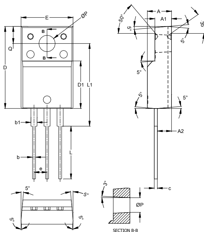
ITO220AB
