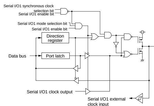
(16) Port P26
