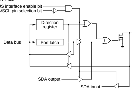
(12) Port P22
