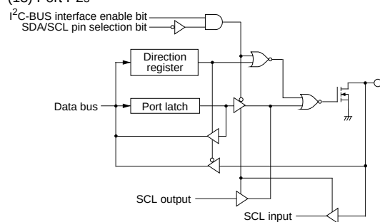
(13) Port P23
