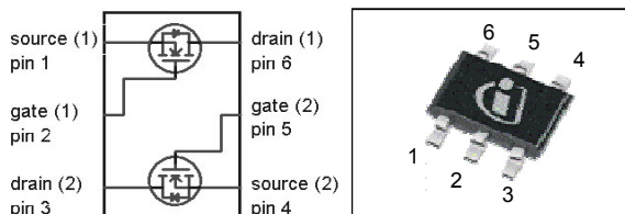
PG-SOT363
