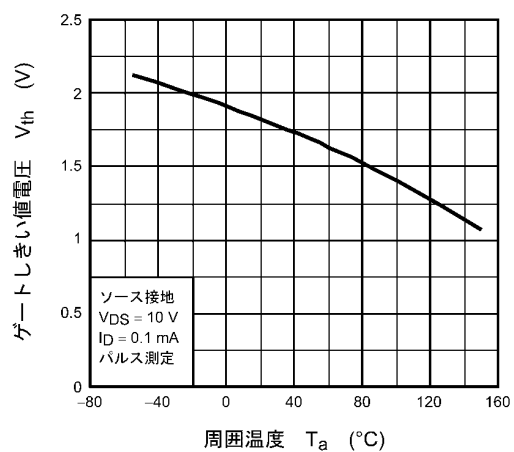
図 8.9 V_{th} - T_a
