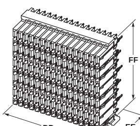
Receptacle (Backplane)
