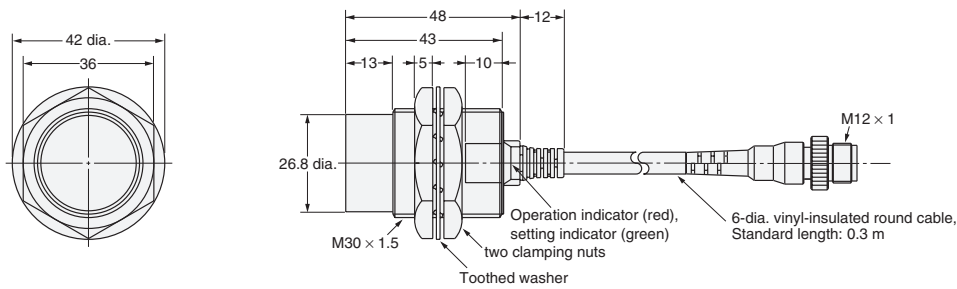
Fig. 34 : E2E-X20MD1-M1GJ
