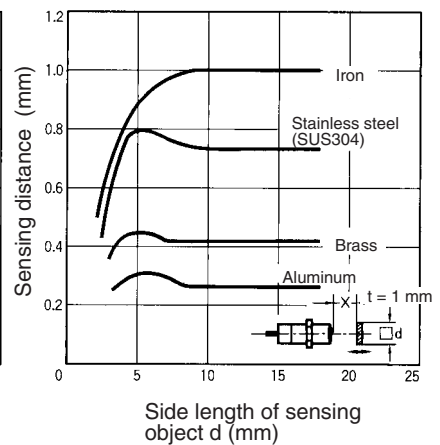
E2E-X1□□ E2E-C1□□
