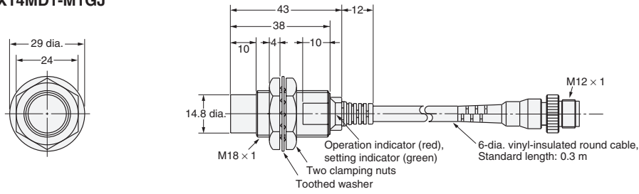
Fig. 32 : E2E-X14MD1-M1GJ
