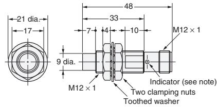
Fig. 20 : E2E-X8MD□-M1(G) E2E-X5ME□-M1/F□-M1
