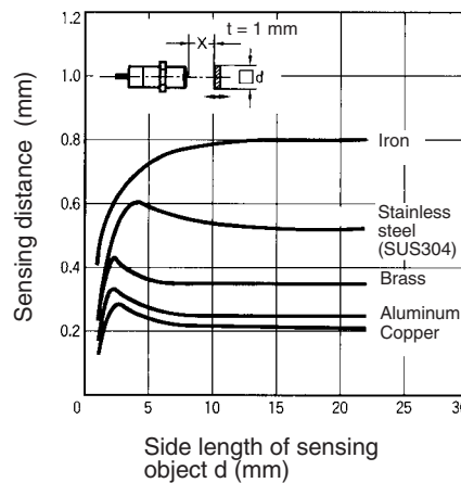
E2E-CR8□□
