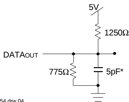
Figure 2. Output Test Load (For t iz , t z , t wz , t ow )
