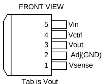
TO263-5L
