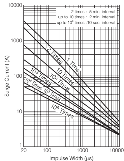
ERZV10D182CS
