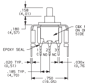
8121SD3_GE SPDT
