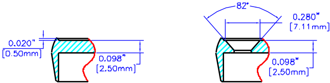
SECTION A-A SCALE 2:1 SECTION B-B SCALE 2:1
