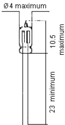
Dimensions : Millimetres
