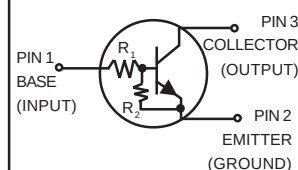
SC-70 / SOT-323
