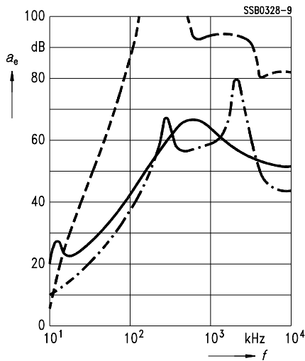
B84299-K66
