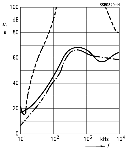
B84299-K67
