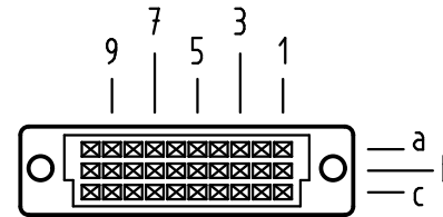
X Kontaktanordnung contact arrangement
