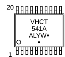
TSSOP-20 SUFFIX DT CASE 948E
