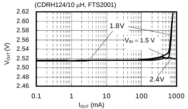
(16) S-8341C25AFT
