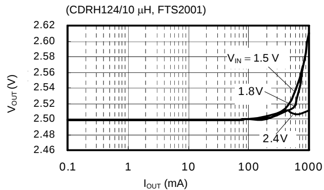
(4) S-8341A25AFT
