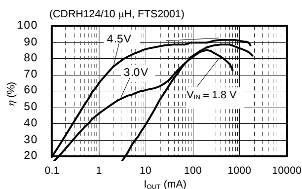
(14) S-8340C25AFT
