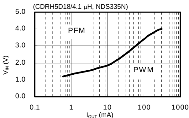
(31) S-8341C25AFT
