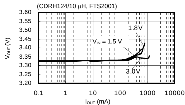
(8) S-8341A33AFT
