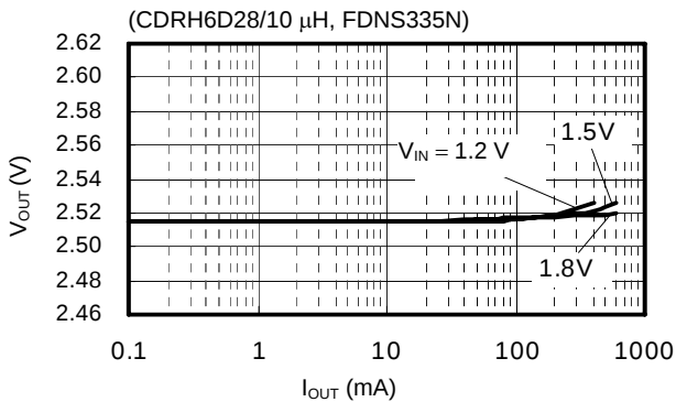
(15) S-8341C25AFT
