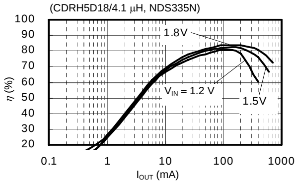
(3) S-8341A25AFT
