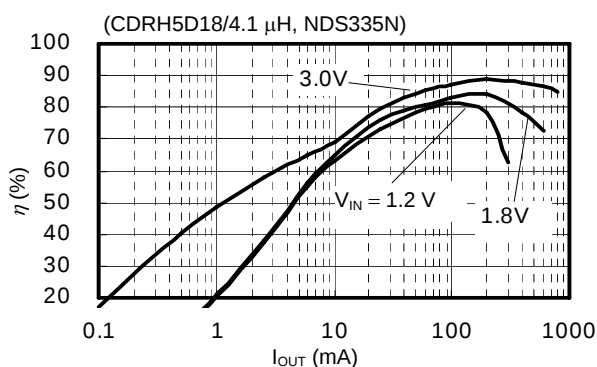
(7) S-8341A33AFT
