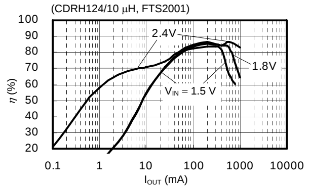
(4) S-8341A25AFT
