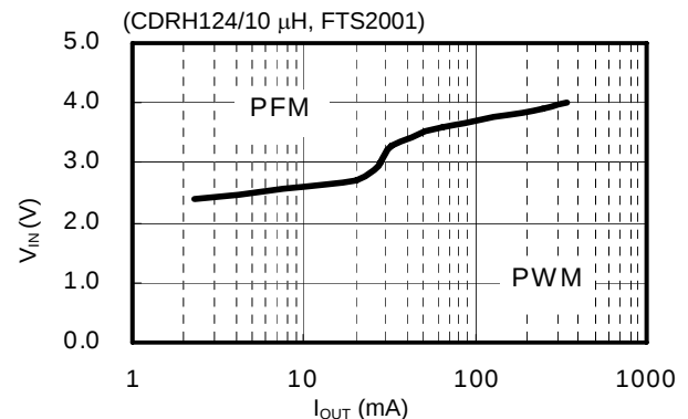
(32) S-8341C25AFT
