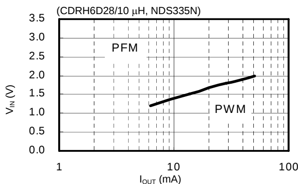
(31) S-8341C25AFT
