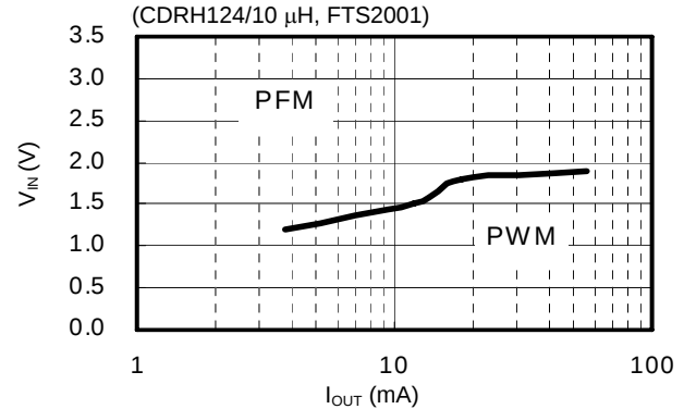
(28) S-8341A33AFT
