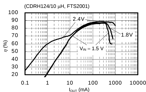
(16) S-8341C25AFT
