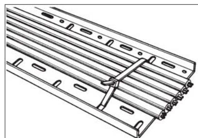
Kabelrännor i praktiken.
