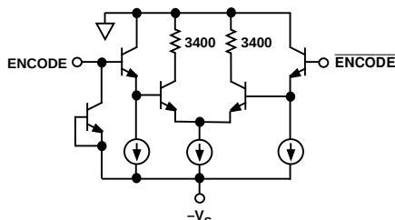
AD9027 Encode Input
