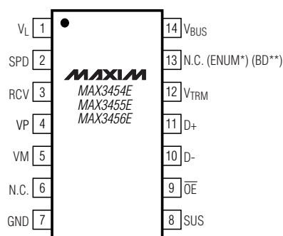
TSSOP
