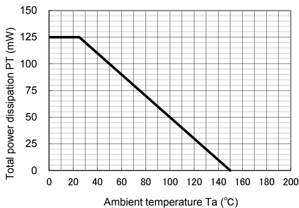
PT - Ta
