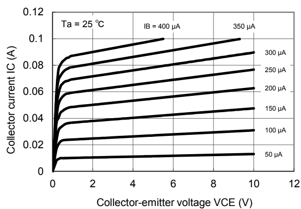
IC - VCE
