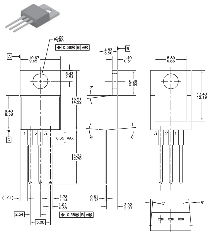
TO-220/TO-220AB
