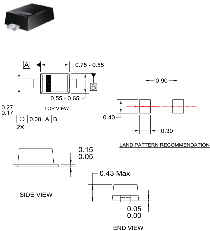
SOD-923
