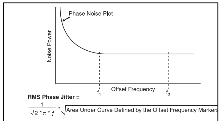
Phase Jitter
