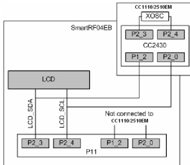
Figure 8: EM LCD connection
