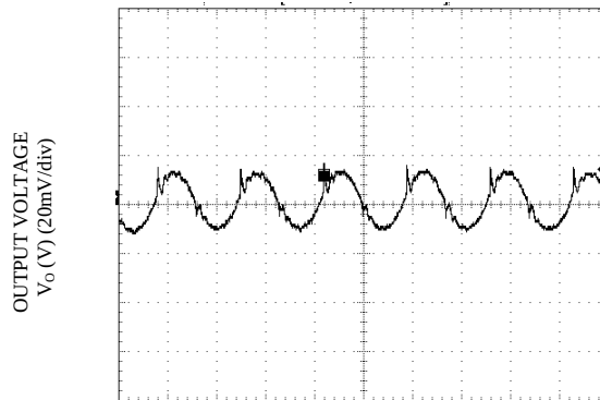
Vin=5V, Vo=1.2V, Io = Io,max
