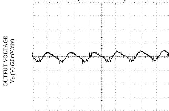
Vin=5V, Vo=0.6V, Io = Io,max
