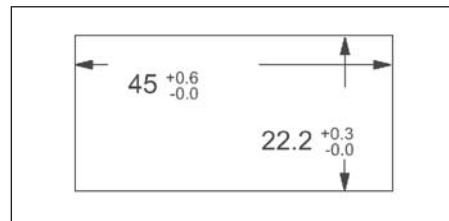
Schalttafelausschnitt ( Angaben in mm )
