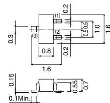
EMT3 (SC-75A) <SOT-416>
