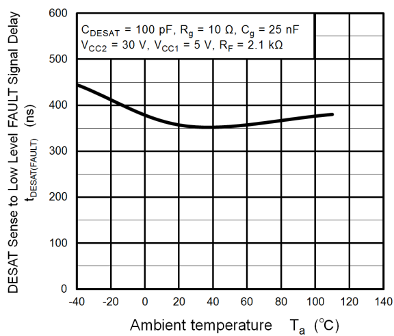
t_{DESAT(FAULT)} - T_a
