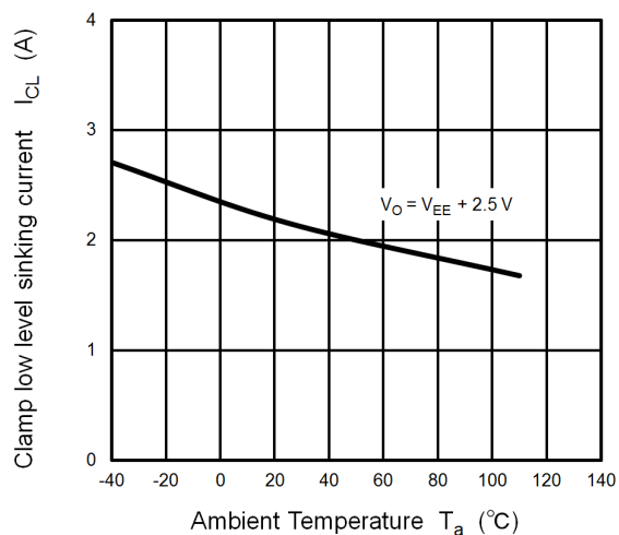
I_{CL} - T_a
