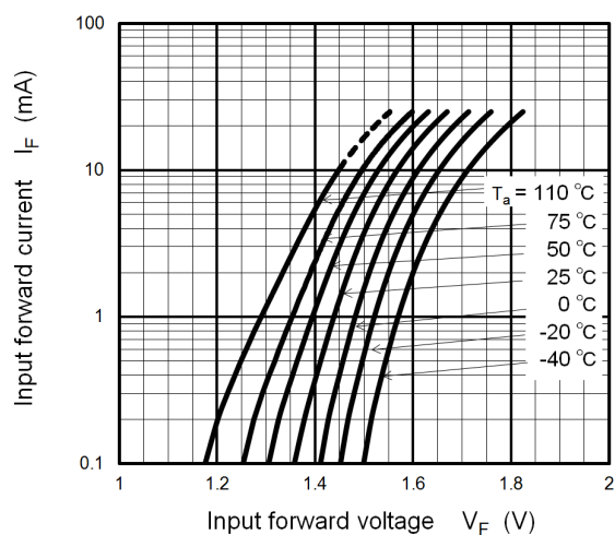
I_F - V_F
