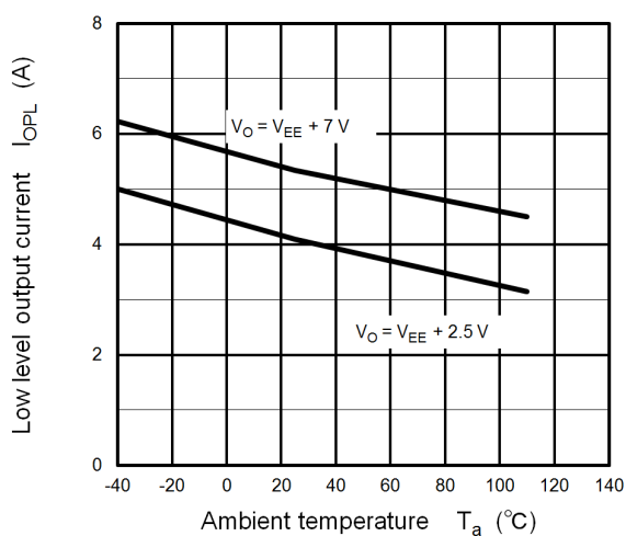
I_{OPL} - T_a
