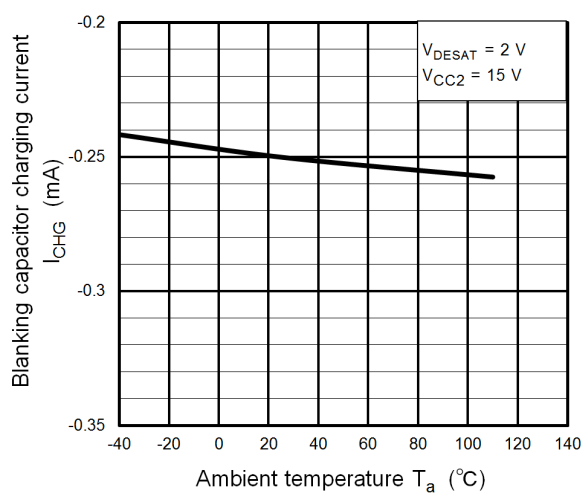
I_{CHG} - T_a
