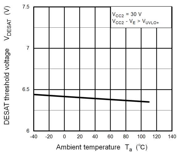
V_{DESAT} - T_a
