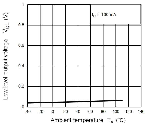
V_{OL} - T_a
