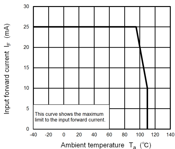
I_F - T_a
