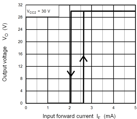
V_O - I_F
