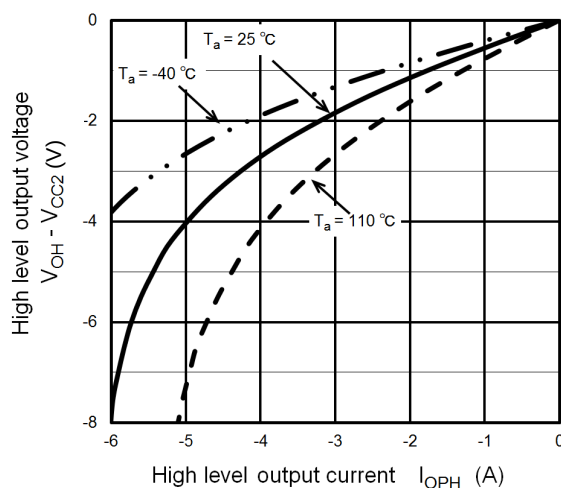
(V_{OH} - V_{CC2}) - I_{OPH}
