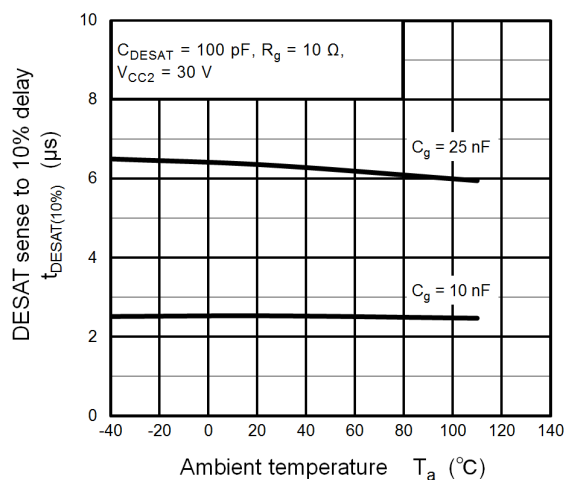
t_{DESAT(10\%)} - T_a
