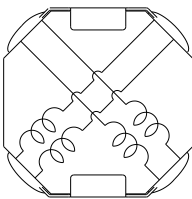
(10μH~47μH)
