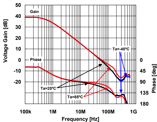
Gain/Phase vs. Frequency (Ambient Temperature) V^+/V^-=\pm 15\text{V} , V_{IN}=0.02\text{V}_{pp} , G_v=40\text{dB} , R_I=50\Omega , R_F=1.98\text{k}\Omega , R_G=20\Omega , C_F=0\text{F} , C_L=10\text{pF} , R_L=500\Omega
