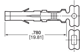
Socket
