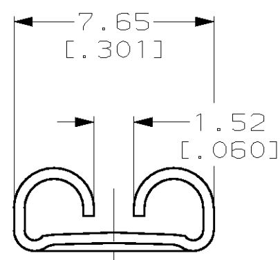
VIEW A-A
