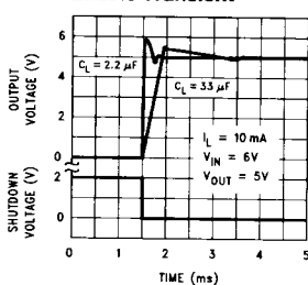
Enable Transient
