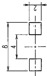
PRINTED CIRCUIT BOARD LAND DIMENSIONS プリント基板ランド寸法
