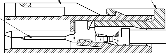
ターミナル及びリテーナー装着状態図 TERMINAL & RETAINER ASSEMBLY DRAWING.
