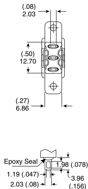
SOLDER LUG
