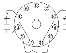
3PDT
