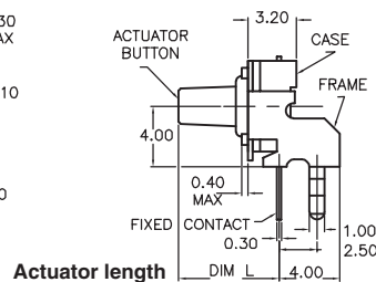
Actuator length
