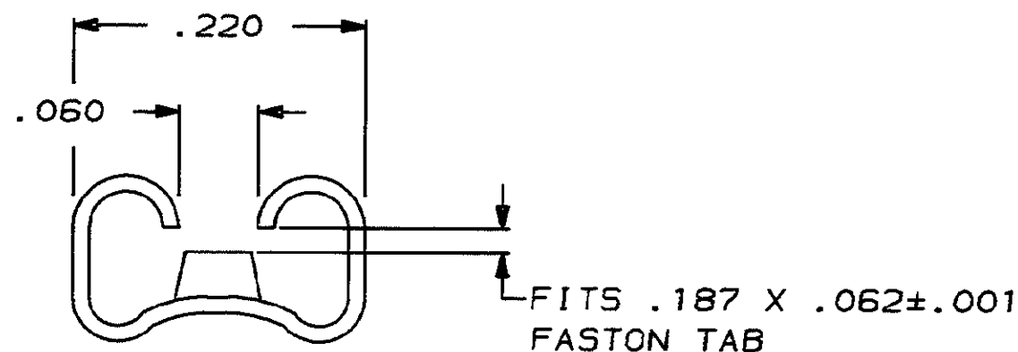
VIEW A-A
