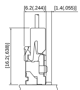
PAF Receptacle + PA Header
