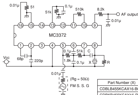
MC3372
