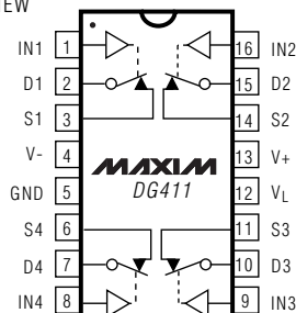
DIP/SO/TSSOP
