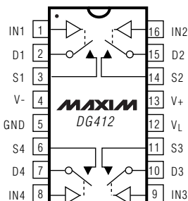
DIP/SO/TSSOP
