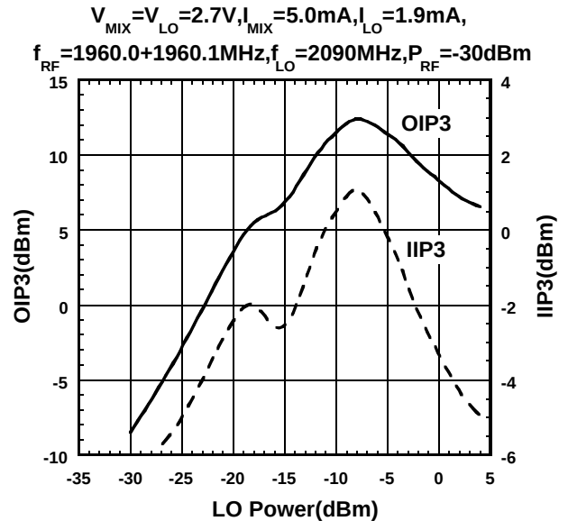
OIP3,IIP3 vs. LO Power
