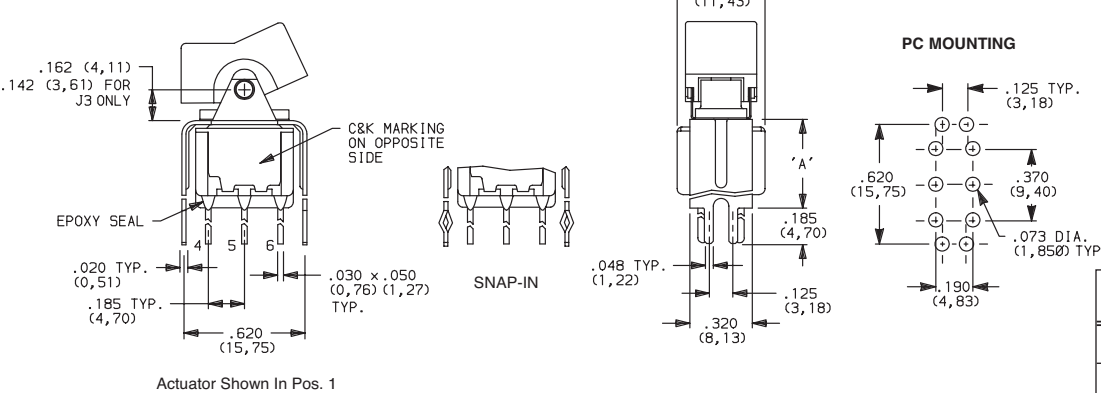
7201J1_BE2 DPDT
